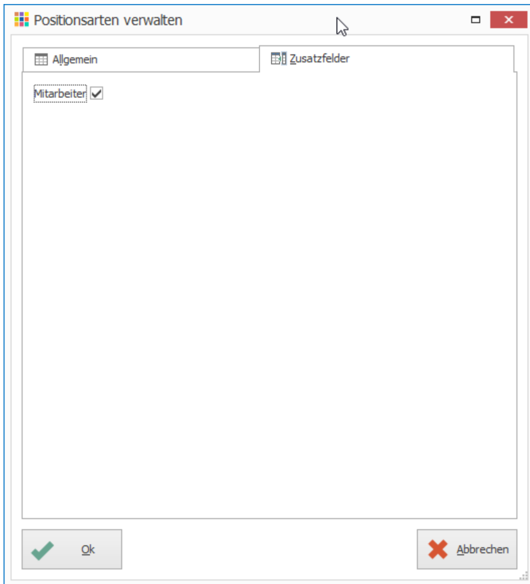
Bild 11: Positionsarten - Zusatzfelder
